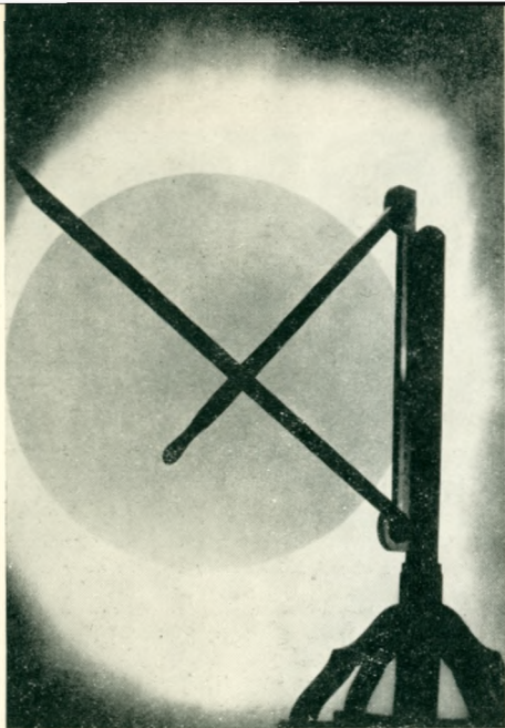
Instrumentarium Mikołaja Kopernika – Triquetrum czyli Instrumentum Paralacticum, najbardziej popularny przyrząd z instrumentów Kopernika, składał się z trzech listew przy pomocy których można było określić kąt między pionem, a badaną gwiazdą, kopia ze zbiorów Muzeum Okręgowego w Toruniu – Oddział Mikołaja Kopernika
