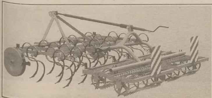
AGREGAT UPRAWOWY KULTYWATOROWY przeznaczony do przedsięwzięcia uprawiania gleby pod zboża, ziemniaki, kukurydzę i buraki. Szerokości robocze od 1,8 m do 4,2 m. Szerokości od 4,6 m do 5,6 m są wyposażone w hydrauliczny układ składania.
