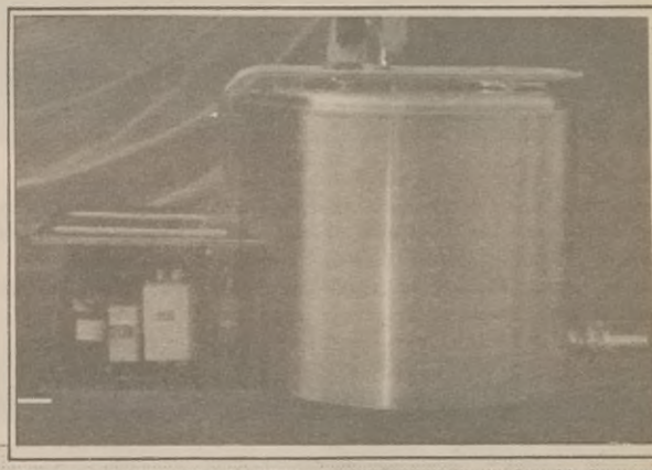
SCHŁADZALNIKI MLEKA TYPU SM: przeznaczone są do schładzania i przechowywania w temp. 4-5°C, mleka. Maksymalny czas schładzania jednego udoju z temp. 35°C do temp. 4°C przy temp. otoczenia 25°C wynosi 2,5 godziny. Oferowane pojemności: * SM-2 poj. 220 l, * SM-3 poj. 300 l, SM-4 poj. 400 l, * SM-6 poj. 600 l, SM-8 poj. 800 l, SM-10 poj. 1000 l, * SM-12 poj. 1200 l.
