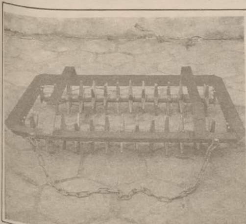
WAŁ KOLCZASTY stosowany za pługiem 3-, 4- lub 5-skbowym.
