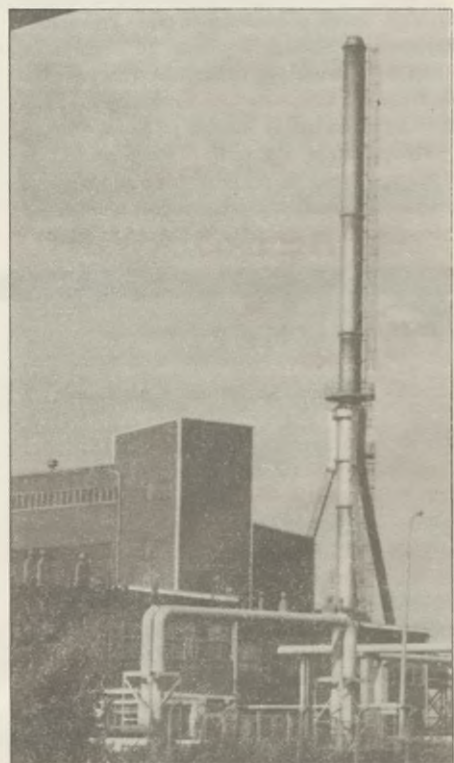
Komin ma 60 metrów wysokości, 190 cm średnicy. Zbudowany jest z blachy o grubości 1 centymetra.
