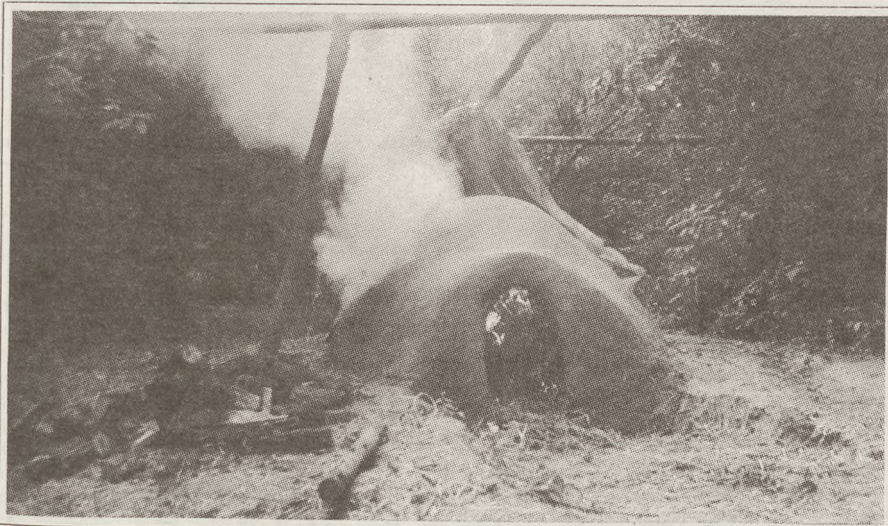
Piec do wypalania ceramiki stojący na terenie rezerwu archeologicznego w Biskupinie w momencie przepalania, które służy wysuszeniu i kontroli jego stanu przed użyciem. fot. Darek Król
