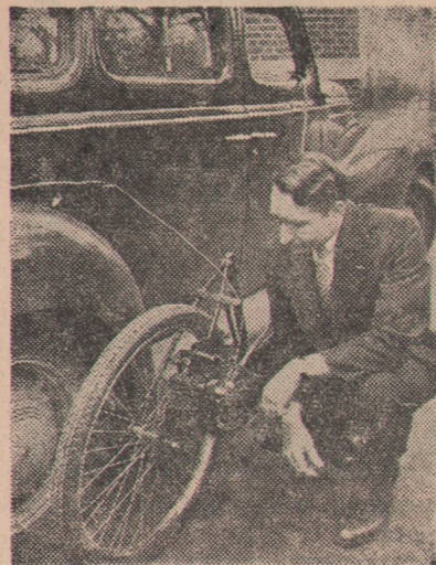
Koło przemocowane do boku samochodu służy instytutowi do przeprowadzenia kontroli nad wymiarem długości trasy przebytej jeszcze przez samochód po użyciu hamulców
