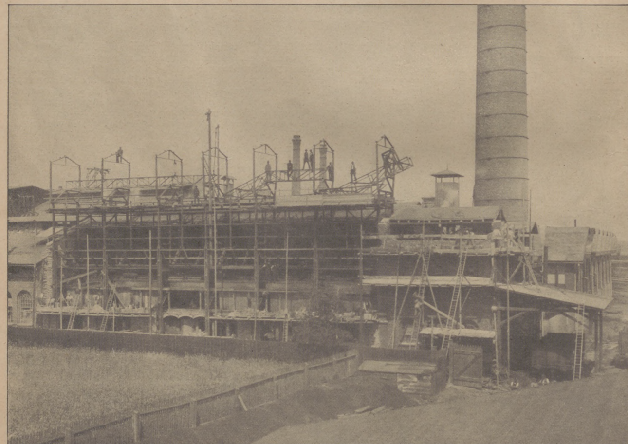
Kohlenbunkeranlage für die Chemische Fabrik der Consol. Alkaliwerke Westeregeln. (F. Eberhardt, Bromberg.)
