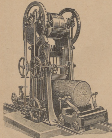
Walzen-Vollgatter.
