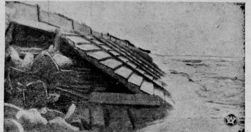
Na zdjęciu widzimy masywną tamę betonową, systemu holederskiego pomiędzy Karwią a Karwińskimi Błotami całkowicie rozbity przez fale morskie.
