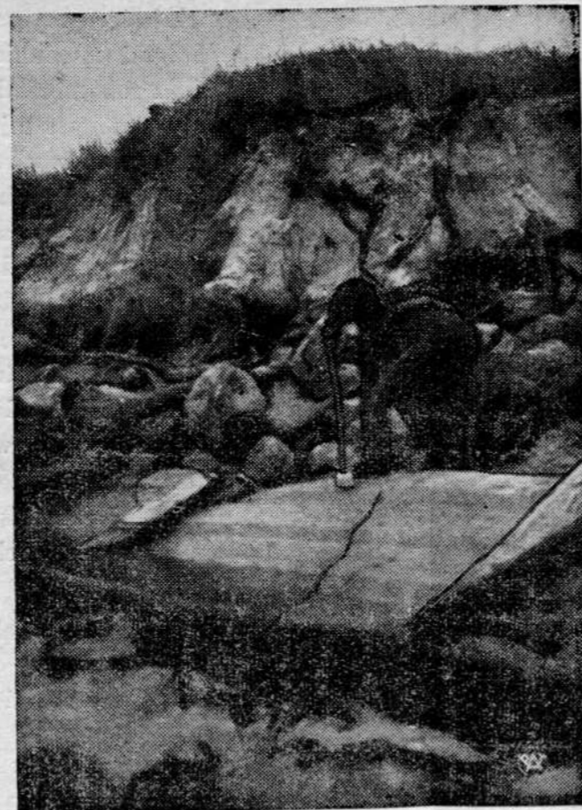
Zniszczona osłona betonowa pod Karwią.
