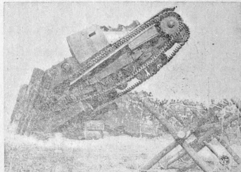
Nowy lekki czołg austriacki pokonuje wszystkie przeszkody
