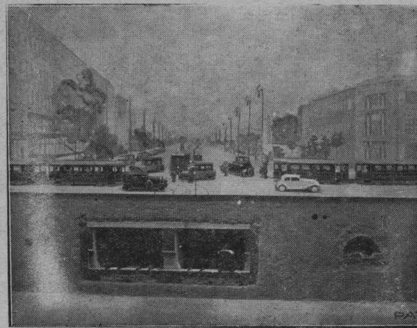
Zdjęcie nasze przedstawia jeden z ciekawych eksponatów, mianowicie panoramę z przekrojem skrzyżowania ulic Nowego Świata i Al. Jerozolimskich. Pod nawierzchnią ulicy widoczny jest tunel nowej linii średnicowej.
