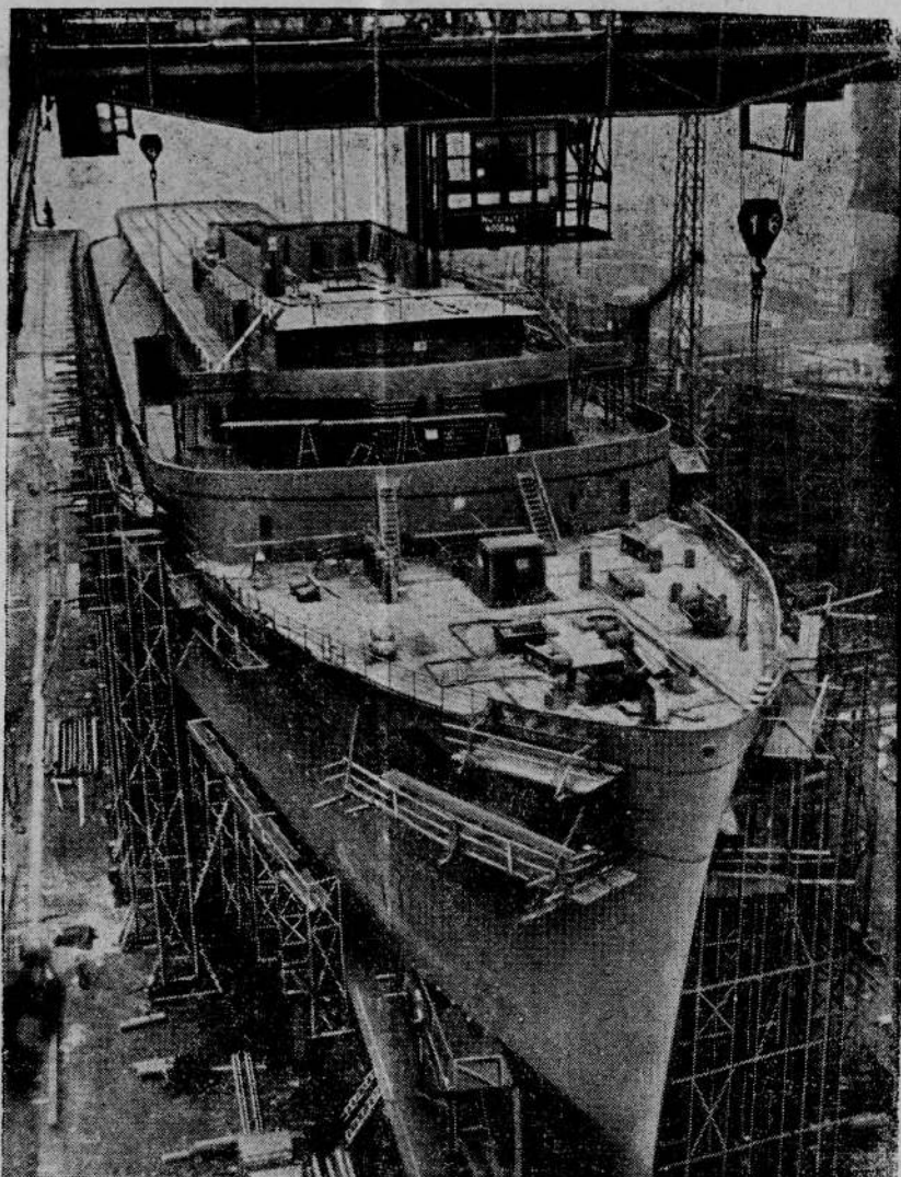
Na stoczni Bloema w Hamburgu ukończona zostanie niebawem budowa okrętu wycieczkowego organizacji „Kraft durch Freude”. Okręt ten pomieścić może 1450 wycieczkowców.
