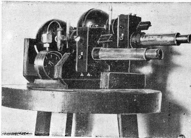
do mierzenia natężenia promieni kosmicznych). Licznik Geigera — przyrząd do badania promieni kosmicznych, który będzie wmontowany w gondole stratostatu.
