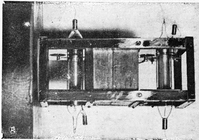
gondole stratostatu „Gwiazda Polski”. Przyrząd nauk., który był używany w poprzednich lotach i który obecnie będzie wmontowany do gondoli (tzw. komory jonizacyjne, służące
