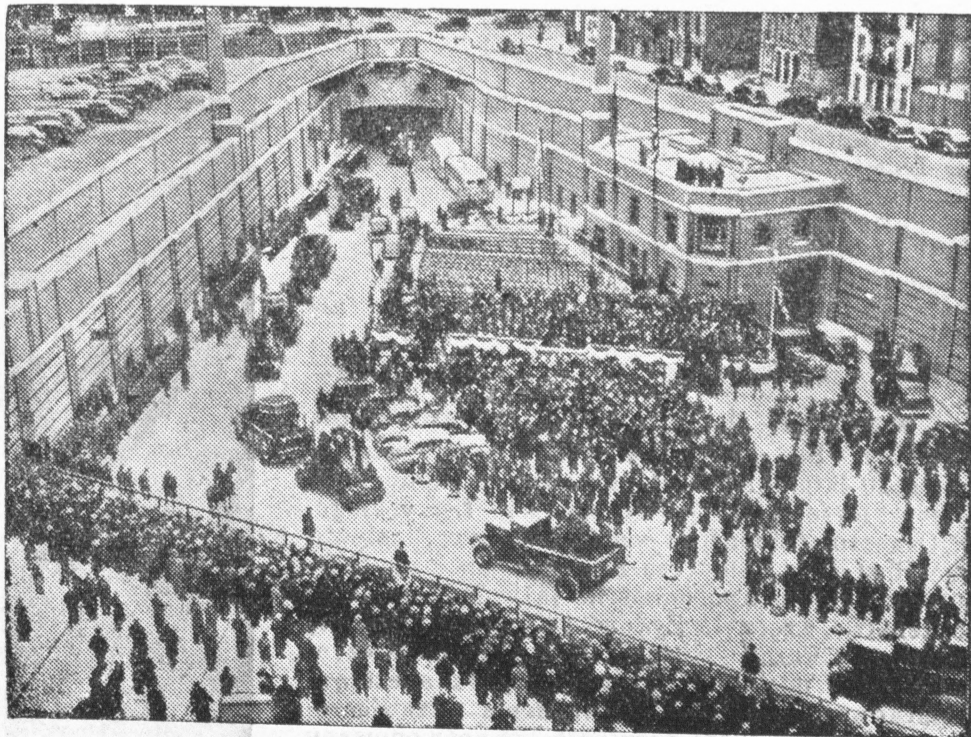
W Nowym Jorku dokonano uroczystego otwarcia nowego wielkiego tunelu im. Lincolna nad rzeką Hudson. Nowy ten stanowi dogodnie połączenie New York City z Weehawken oraz New Jersey. Koszt budowy tego wielkiego tunelu, będącego chlubą inżynierii amerykańskiej, wyniósł zawrotną sumę 75 milionów dolarów. — Na zdjęciu korowód samochodów, wjeżdżających do nowego tunelu w dniu otwarcia.
