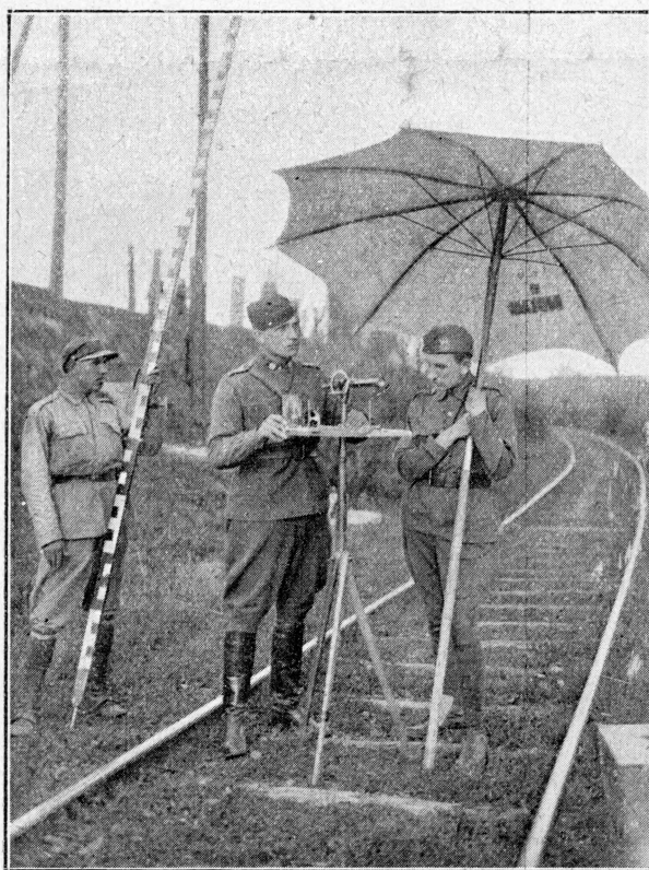
Topograf przy pracy na linii kolejowej
