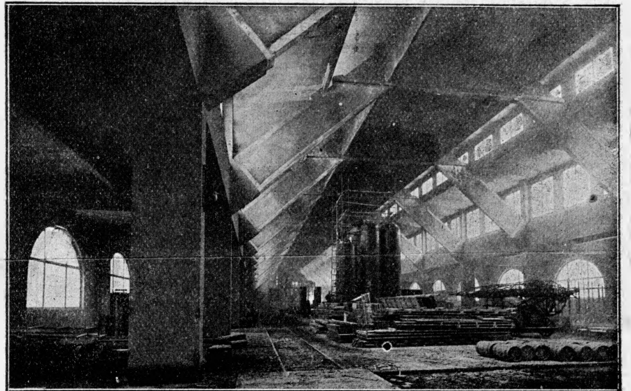
Wnętrze hali ciężkiego przemysłu na P. W. K. W głębi dużych rozmiarów ekspozyty wielkich odlewni żelaza i budowy maszyn.
