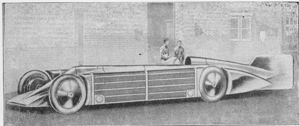
Maszyna majora Sengrave, „Złota strzala” ma osiągnąć fantastyczną szybkość 230 — 240 mil. na godzinę. Projektował maszynę inżynier Irving.
