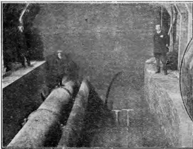
Budowa najwyższego węzła pod ul. Krasieńskiego. Ma on odciążać kolektor bielański.
