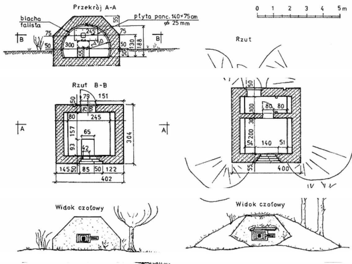
1. Typowe stanowiska bojowe: 1. Pozycji Piłskiej na 1 MG oraz 2. Pozycji Szczycieńskiej w Spychowie. Pomiar i oprac. J. Miniewicz, 1975
